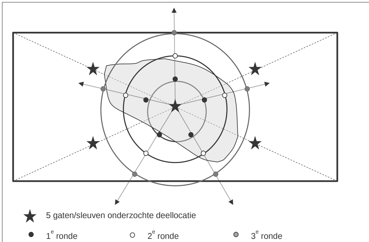
figuur 5: visuele voorstelling afperking via proefgaten/boringen
