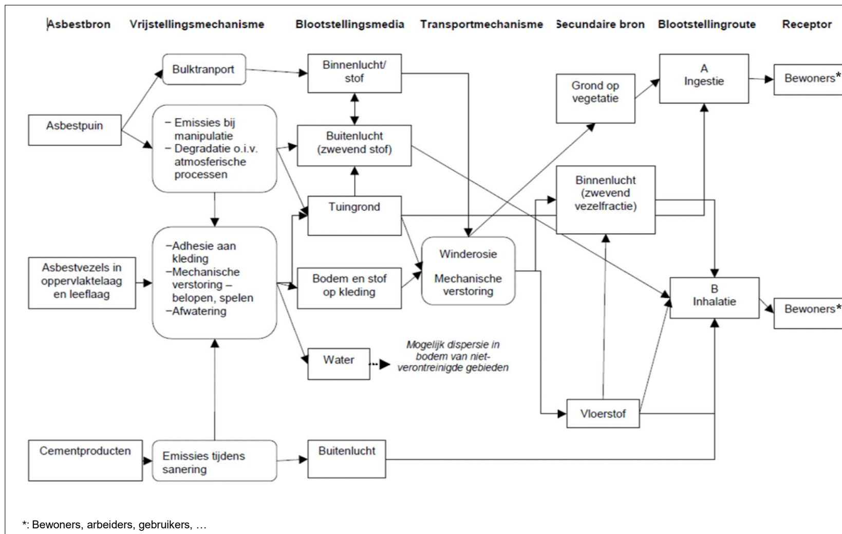
figuur 7: CSM asbest – blootstellingswegen
