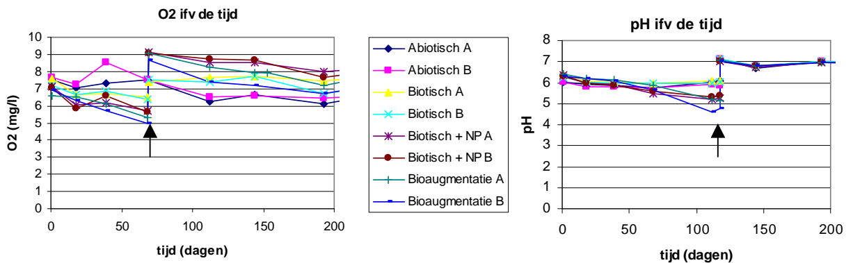
Figuur 2: Evolutie opgeloste zuurstof (toevoeging extra zuurstof aangeduid met pijl) en pH (pH-correctie aangeduid met pijl) in de tijd – batchtest.
