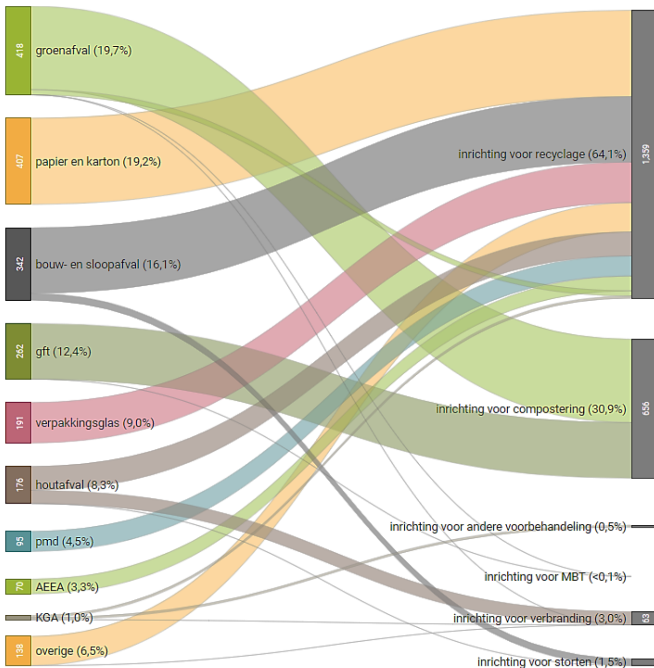
Figuur 14: Stroomdiagram met aanduiding van de inrichting voor verwerking per fractie van het selectief ingezameld huishoudelijk afval in het Vlaamse Gewest in 2017 (hoeveelheden in kton).
