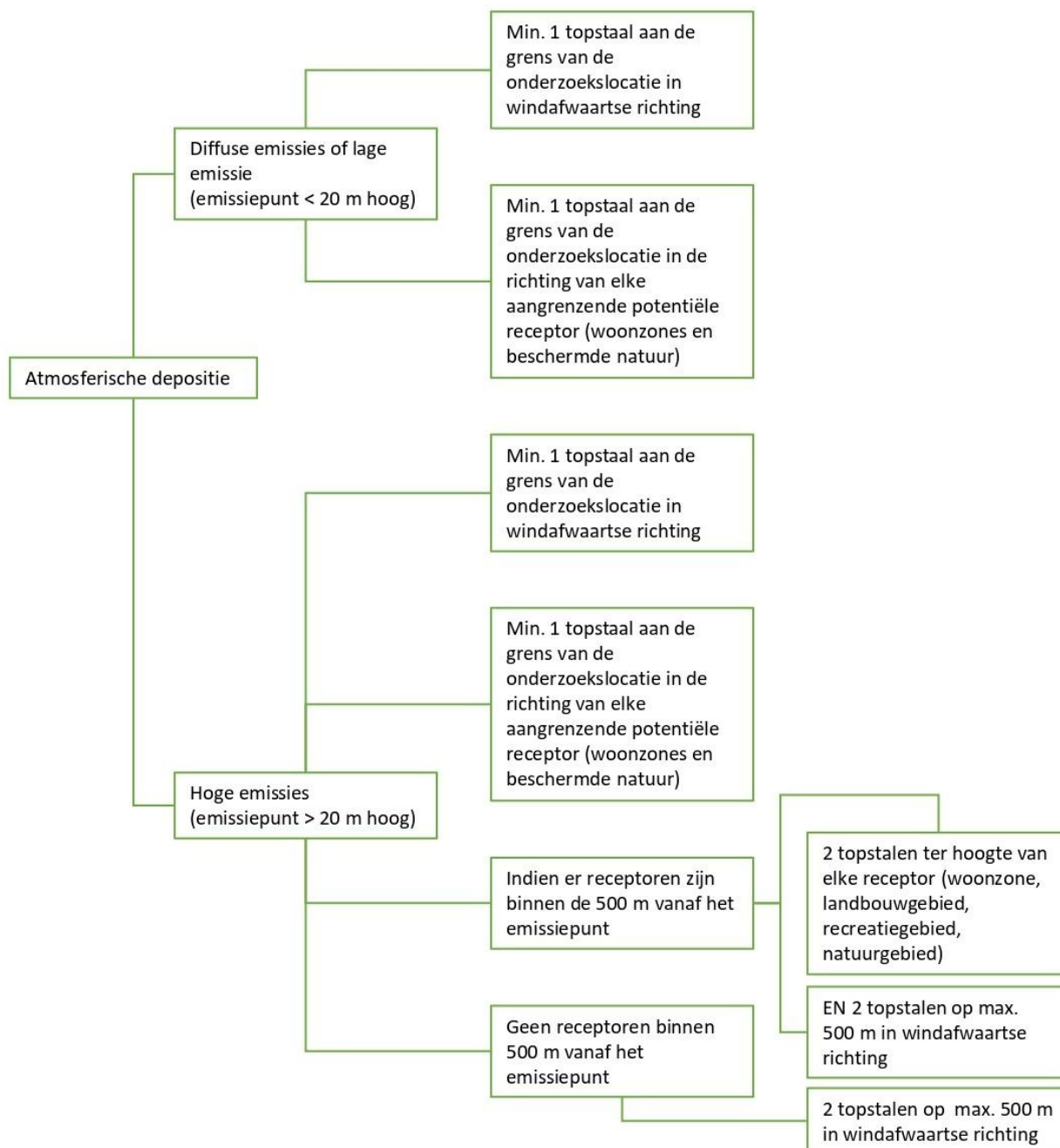
figuur 3: stroomschema bijkomende staalnames en analyses.
