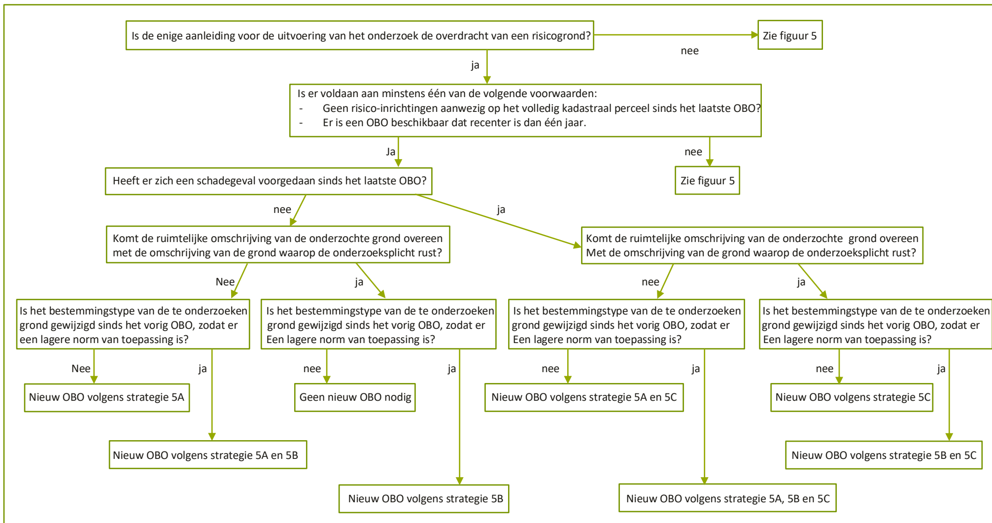
figuur 4: toepassing van bemonsteringsstrategie 5 – uitgezonderd bemonsteringsstrategie 5E
