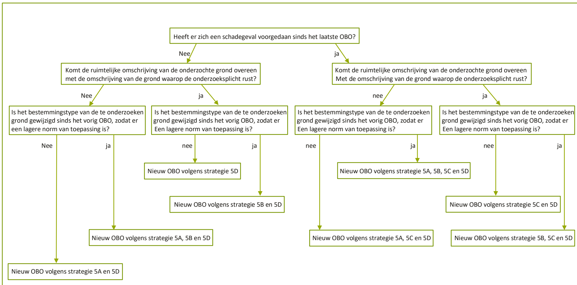
figuur 5: toepassing van bemonsteringsstrategie 5 als er op de onderzoekslocatie nog risico-inrichtingen aanwezig waren sinds het vorige oriënterend bodemonderzoek (OBO) op het volledige kadastrale perceel – uitgezonderd bemonsteringsstrategie 5E
