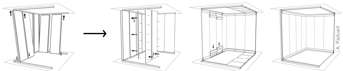
Figuur 57: Preassemblage van dynamische wandpanelen die op de bouwwerf worden afgewerkt
