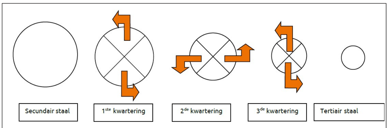
Figuur 2. Visuele weergaven van de methode 'menging, kwartering en reducering'
